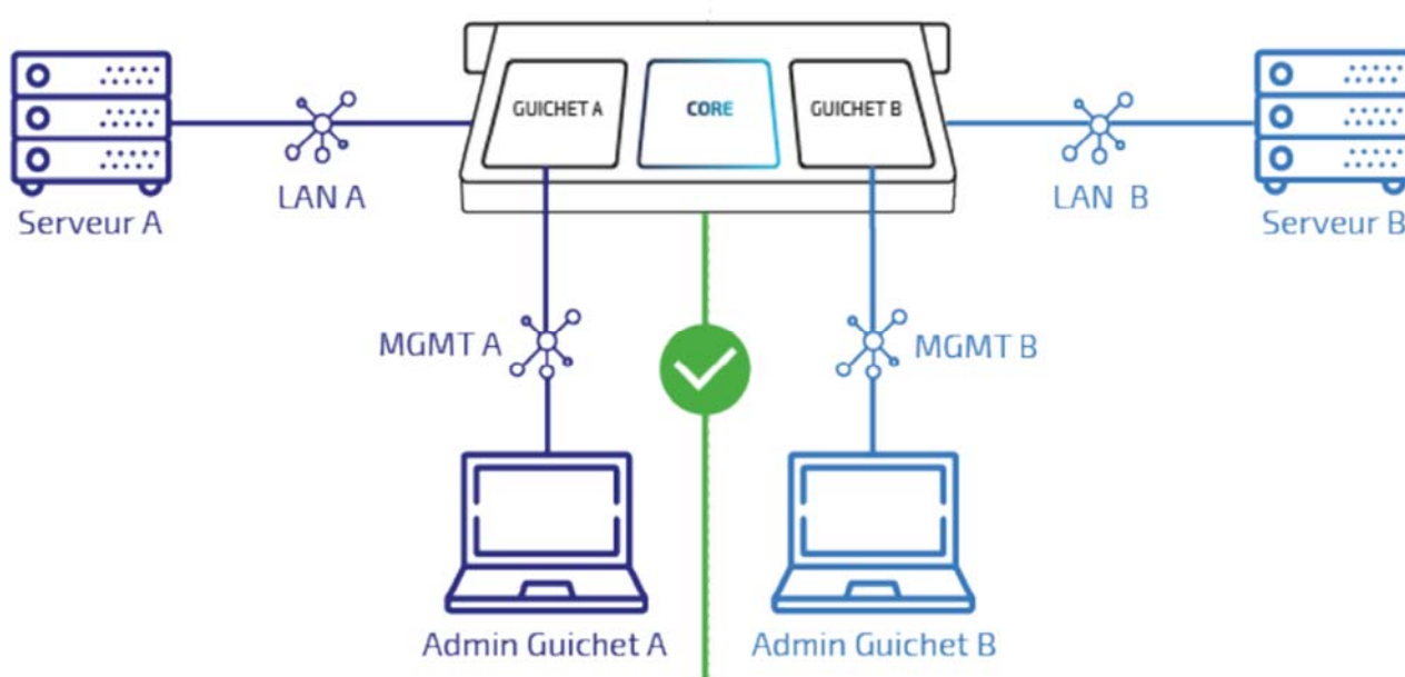
Figure 1 - Architecture Produit.
